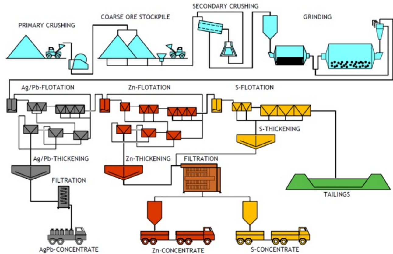
Bild 1. Utvinningsprocess hos Sotkamo Silver
