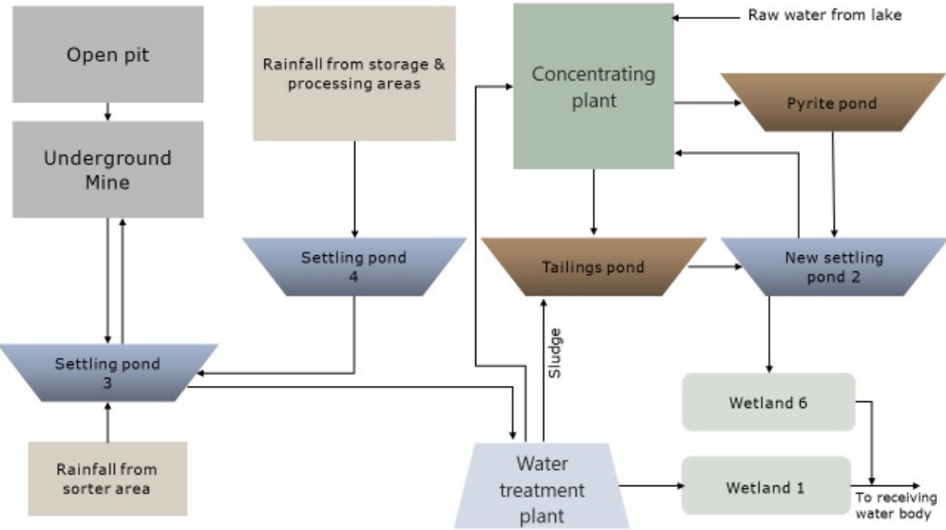
Bild 5. Silvergruvans vattenbalans.
