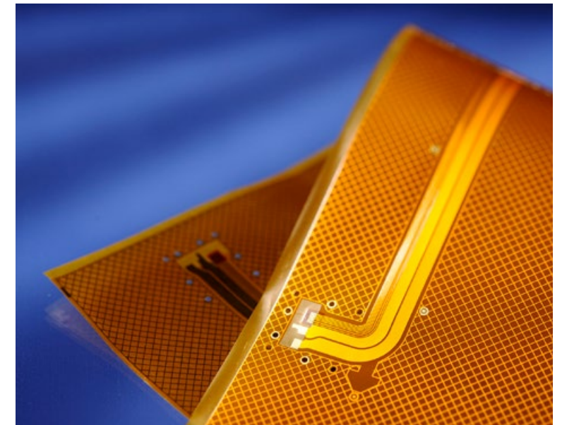
Bild 11. Kretskort tillverkade med en kopparkloridlösning
